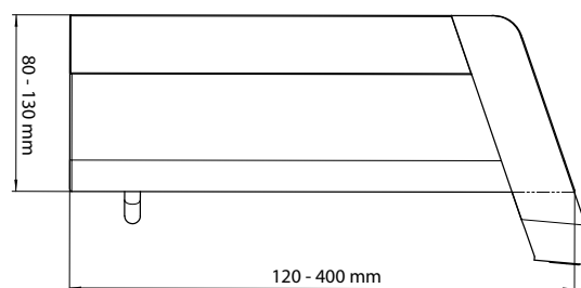
SEITENANSICHT
